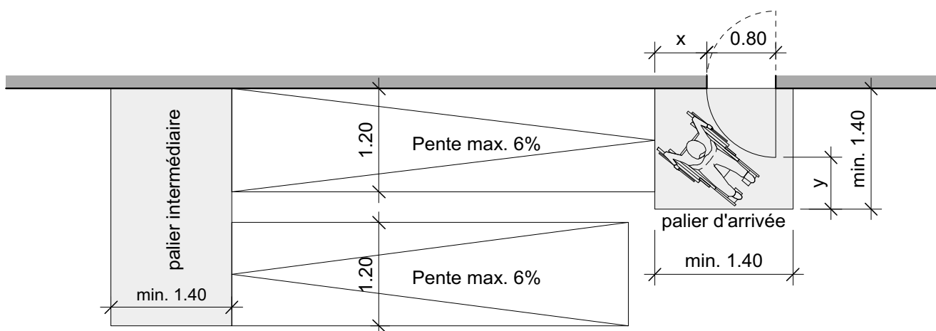
Exemple: rampe avec palier intermédiaire
