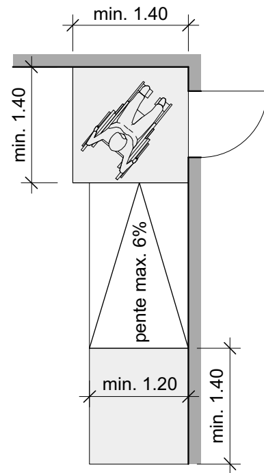
Exemple: rampe avec arrivée de côté
