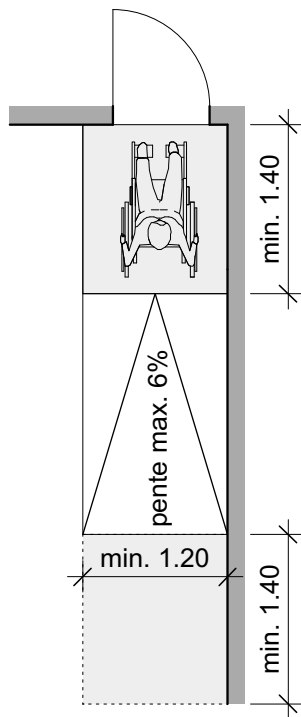
Exemple: rampe avec arrivée droite
